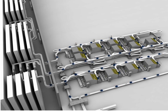
Layout système
